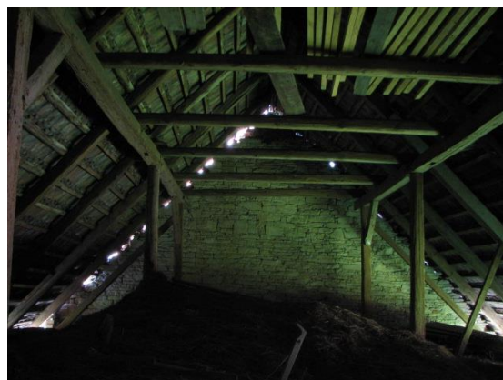
21. Pohled na krov nad komorou a chlévy. Hambalkový krov s dvojicí stojatých stolic.
