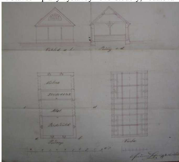
7. Stavební plány výstavby nové stodoly, nedatováno.
